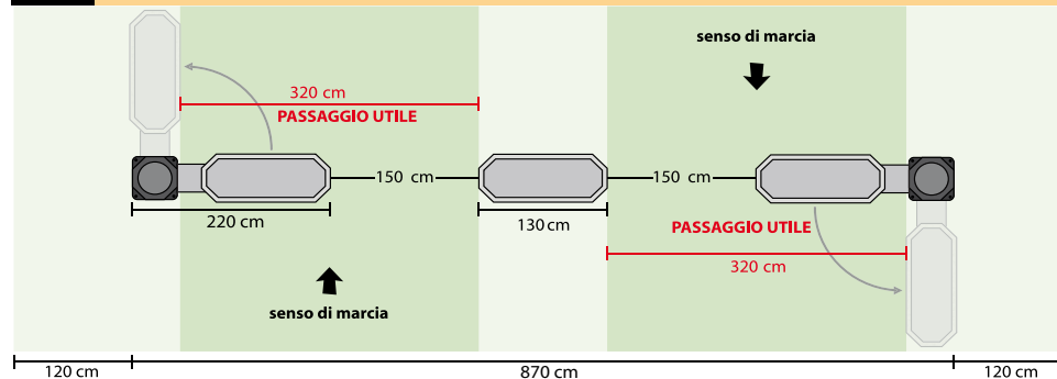
8 Fissa centrale + mobili laterali.
