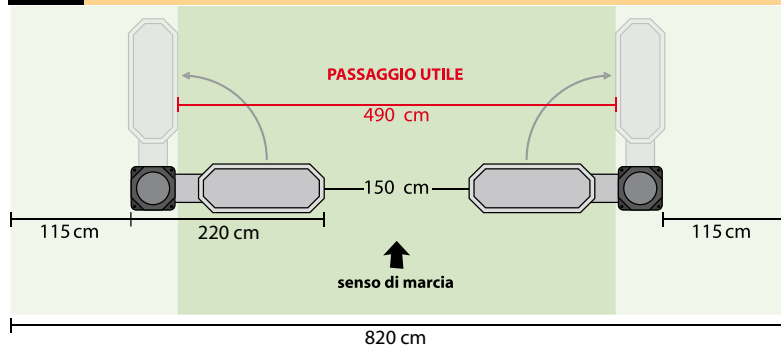
2 Doppia fissa laterale + mobile laterale.
