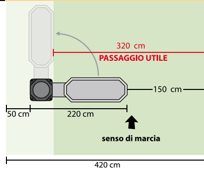
8 Fissa centrale + mobili laterali.
