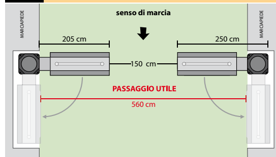
4 Doppia mobile con carrello e incasso nel marciapiede.
