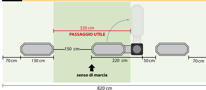
3 Mobile centrale e fisse laterali.
