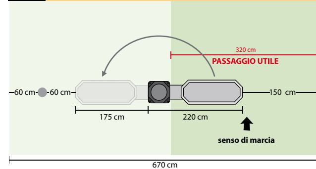
7 Barriera a rotazione 180°.
